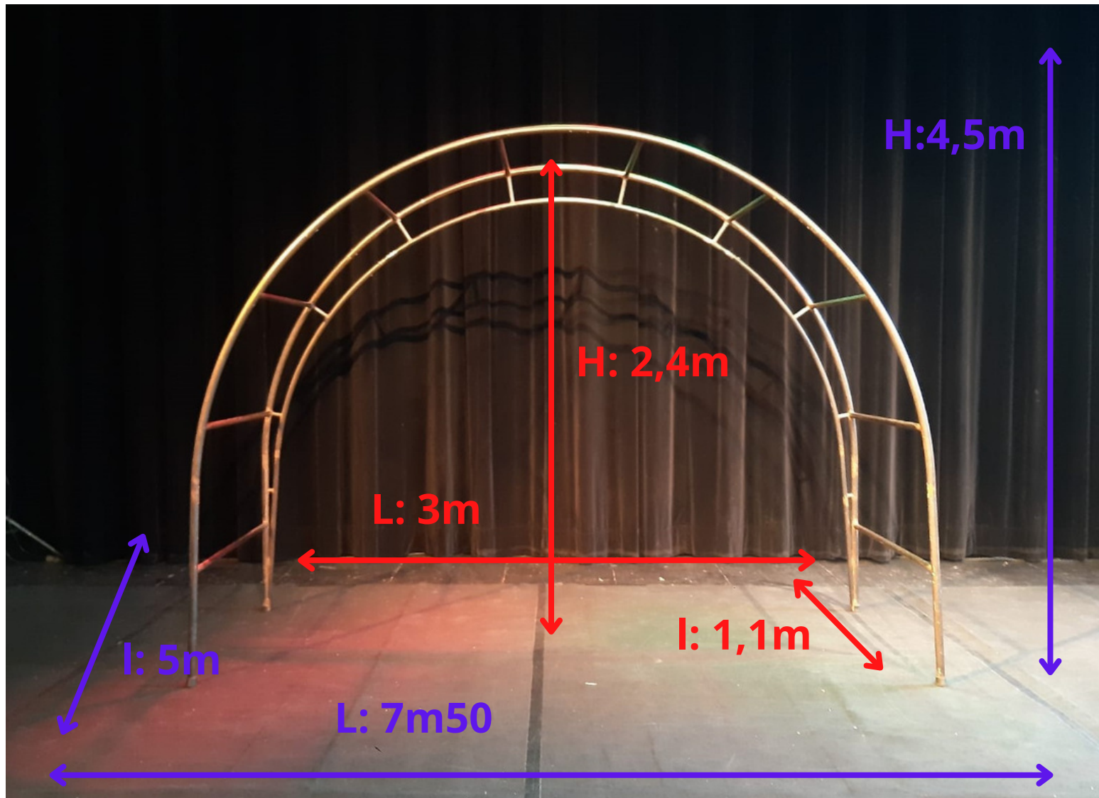
ARCHE structure auto-portée
